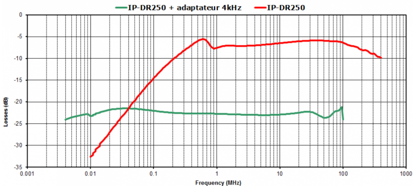
S21 de la pince d'injection induant le JIG de calibration
